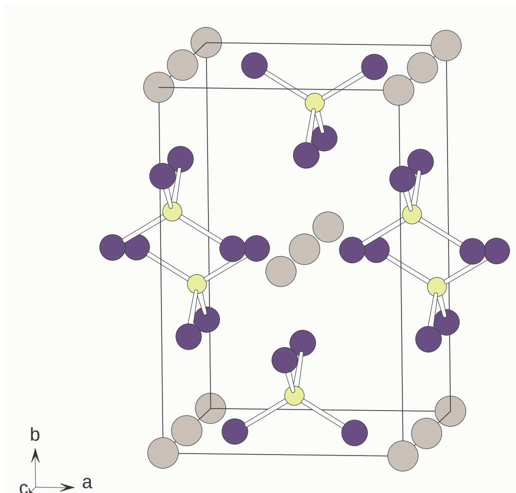
Abb. 1: Elementarzelle einer ABX_4 -Kristallstruktur
