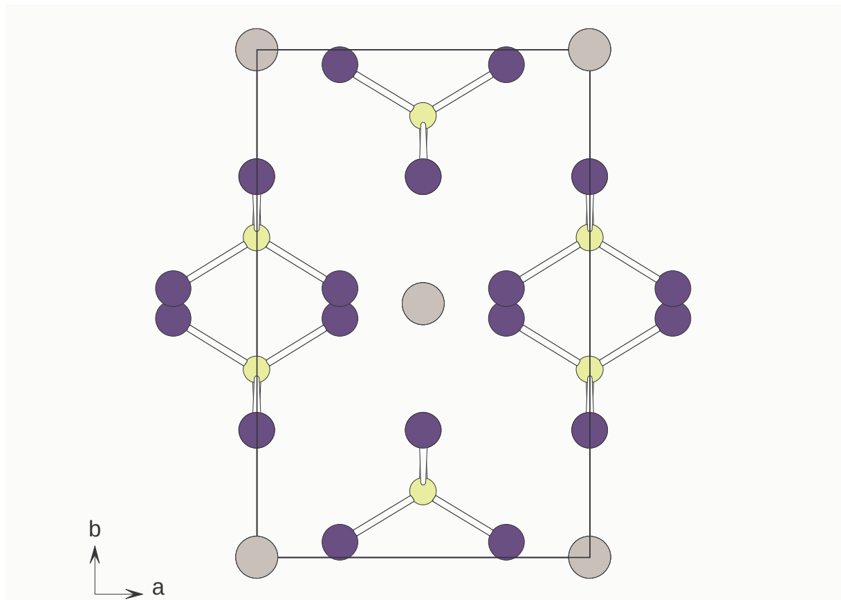
Abb. 4: Projektion der Kristallstruktur in Richtung [001]
