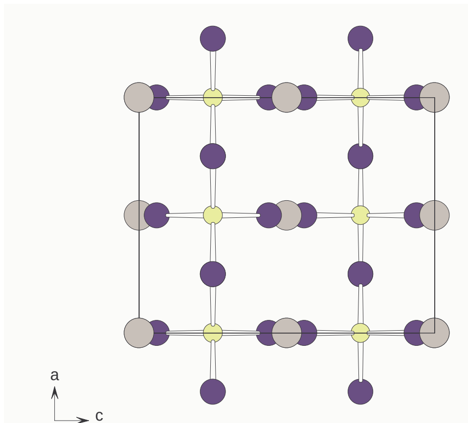
Abb. 3: Projektion der Kristallstruktur in Richtung [010]
