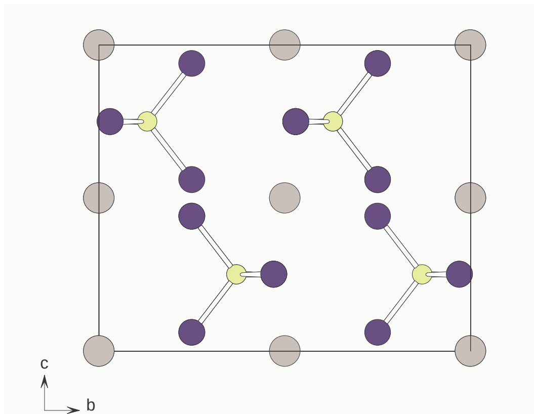
Abb. 2: Projektion der Kristallstruktur in Richtung [100]
